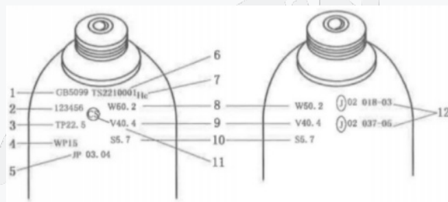
图气瓶钢印示图
