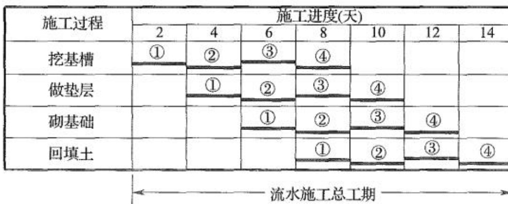
图 3.4.1 流水施工横道图表示法
